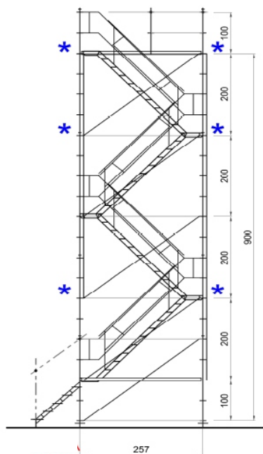
PROSPETTO FRONTALE
