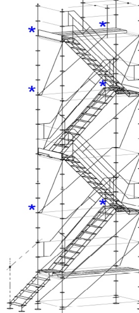
ASSONOMETRIA
